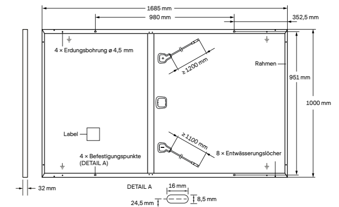
Abb. 2: Außenmaße (in mm) und Komponenten für Q.PEAK DUO-G5.1, Q.PLUS DUO-G5.1, Q.PEAK DUO-G5.3 und Q.PLUS DUO-G5.3
