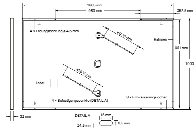
Abb. 1: Außenmaße (in mm) und Komponenten für Q.PEAK DUO-G5, Q.PEAK DUO BLK-G5, Q.PLUS DUO-G5, Q.PLUS DUO BFR-G5, Q.PEAK DUO-G5.2, Q.PEAK DUO BLK-G5.2, Q.PLUS DUO-G5.2 und Q.PLUS DUO BFR-G5.2
