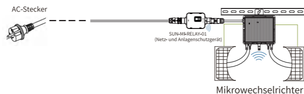
Schaltplan
