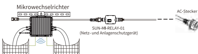
Schaltplan
